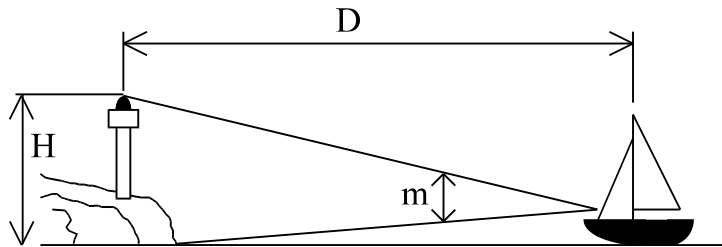
Abb. 10: Prinzip der Vertikalwinkelmessung
