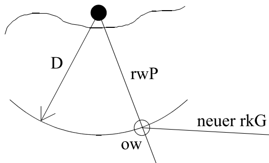
Abb. 11: Standlinie durch Vertikalwinkelmessung
