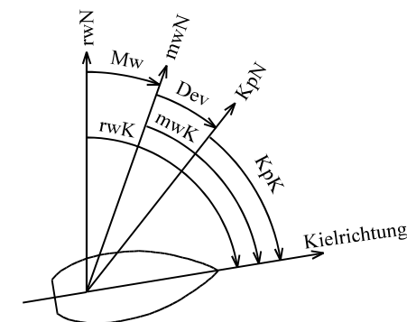
Abb. 5: Missweisung und Deviation
