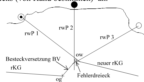
Abb. 14: Kreuzpeilung
