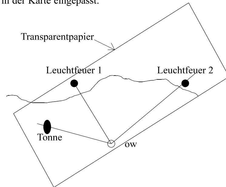
Abb. 19: zwei Horizontalwinkel: Grafische Lösung
