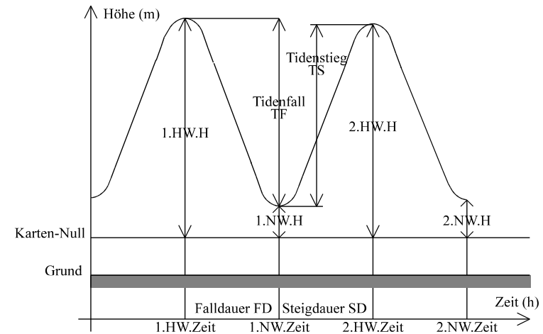
Abb. 23: Gezeiten Begriffe
