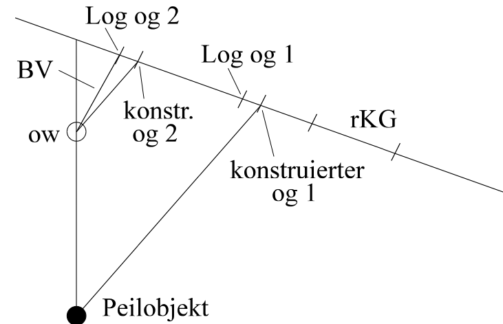
Abb. 17: berechneter und konstruierter og
