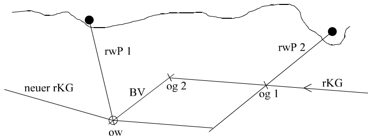
Abb. 16: abgestumpfte Doppelpeilung
