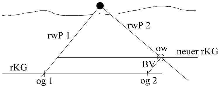
Abb. 15: Doppelpeilung
