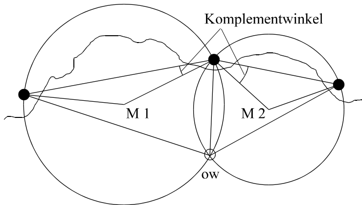
Abb. 20: zwei Horizontalwinkel konstruiert
