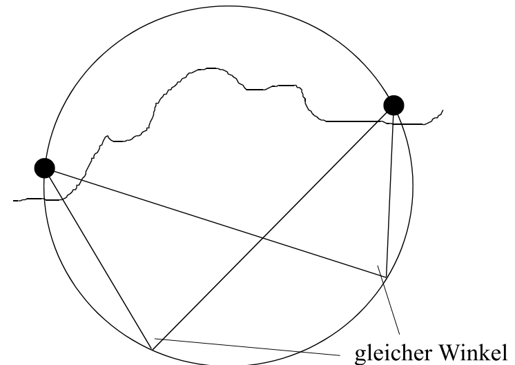
Abb. 12: Standlinie durch Horizontalwinkel
